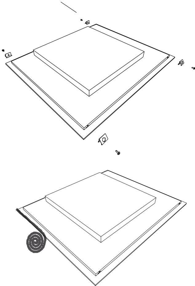
Support de montage pour plan de travail
