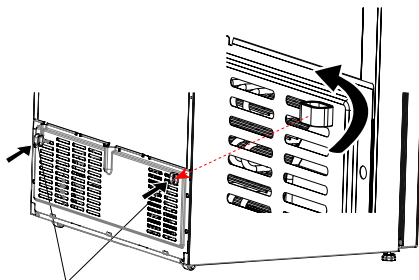
Entretoises pour le réglage de distance
