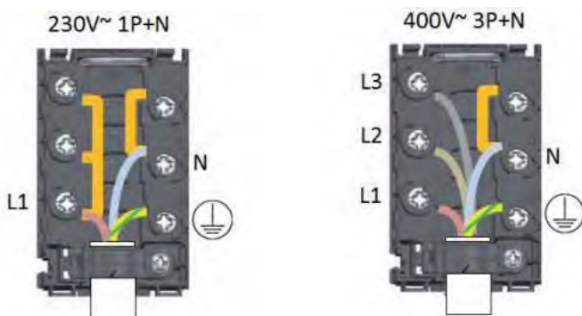
Branchement d'usine
